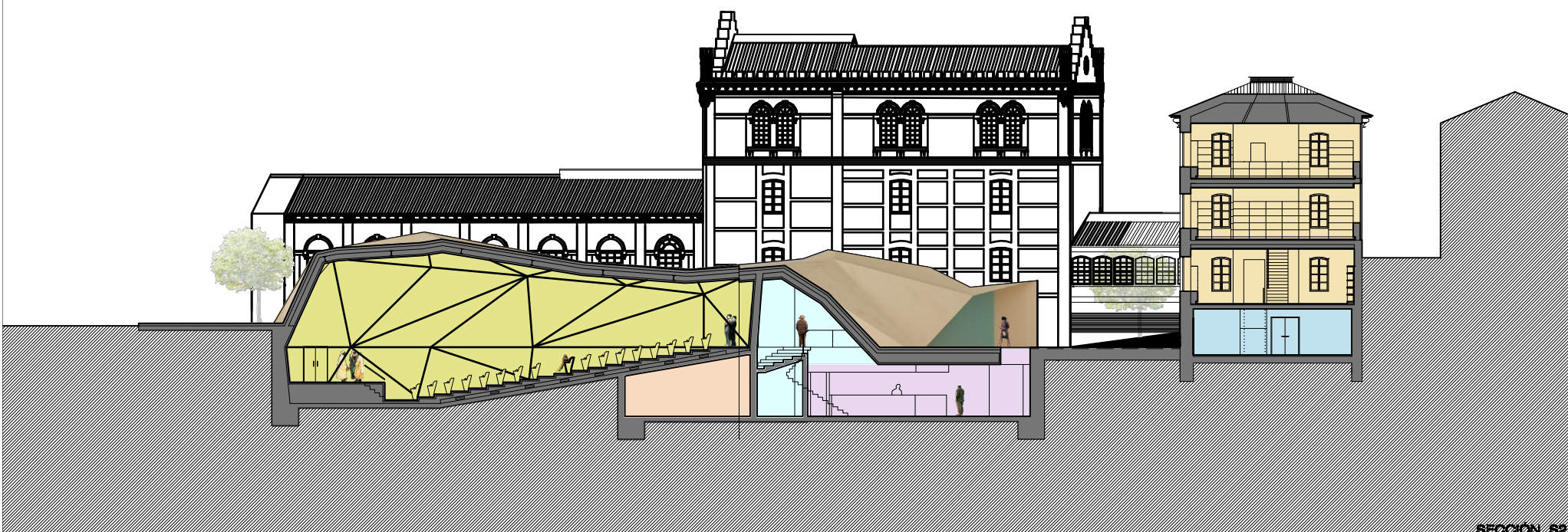
SECCIÓN. S2
