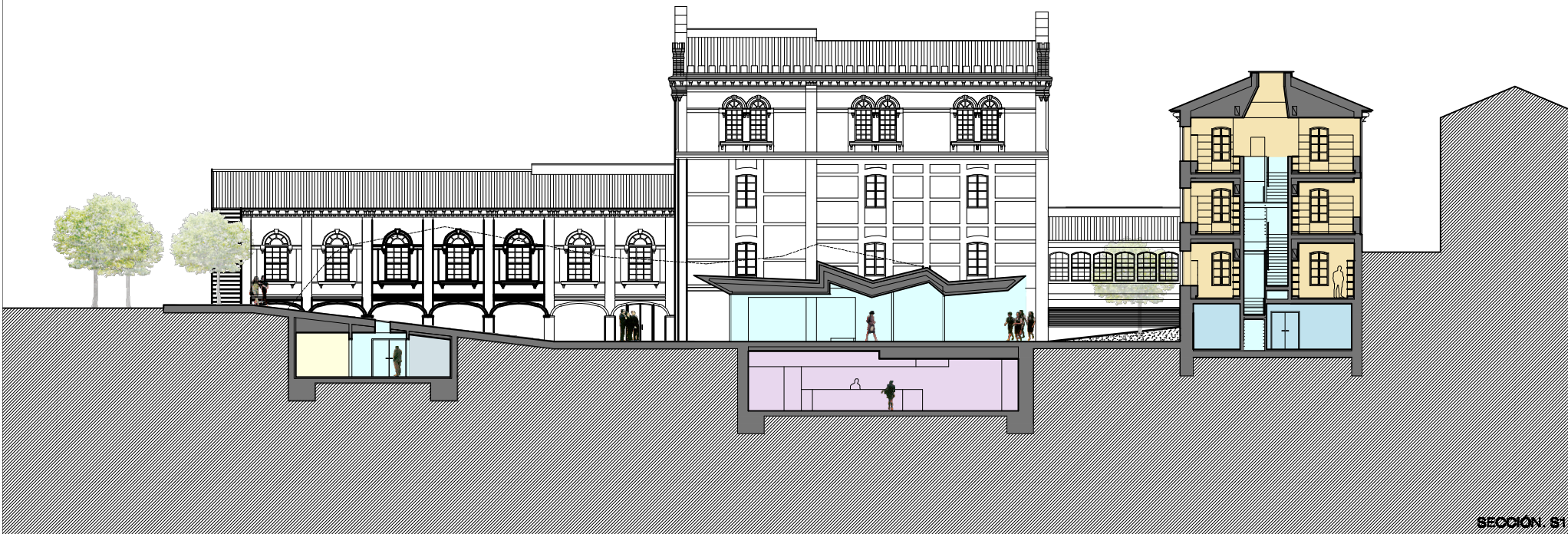
SECCIÓN. S1
