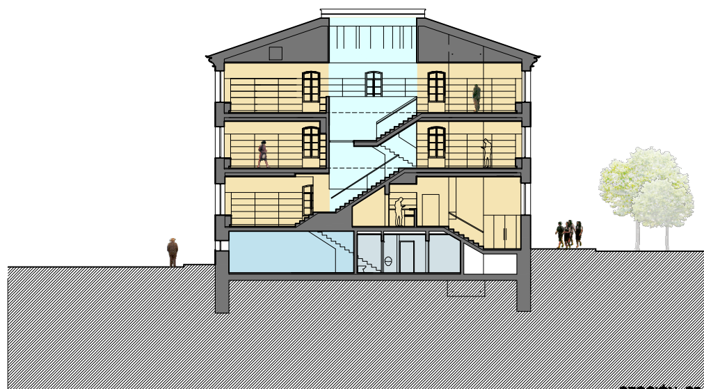
SECCIÓN. S3
